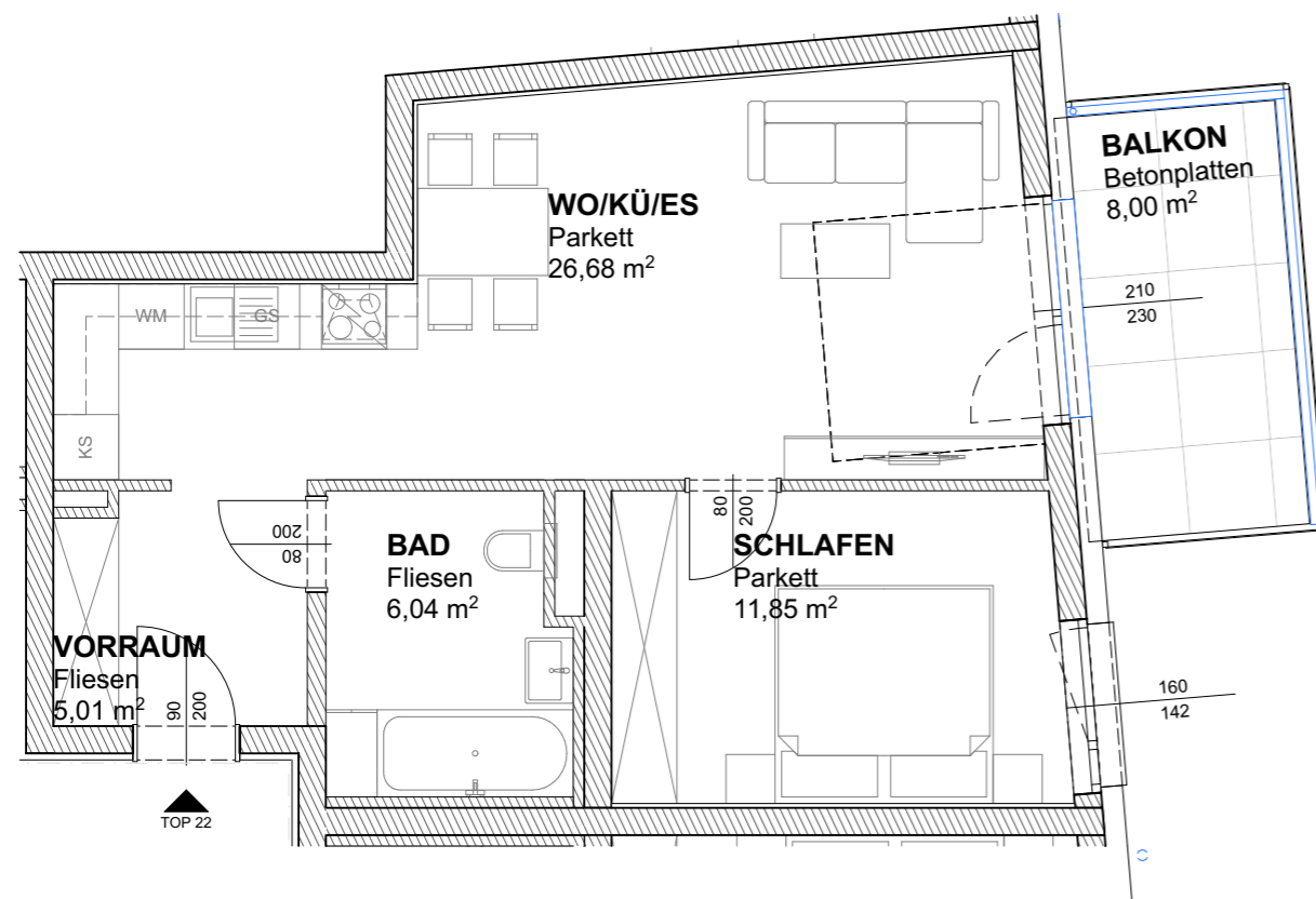
GRUNDRISS | M 1:75
