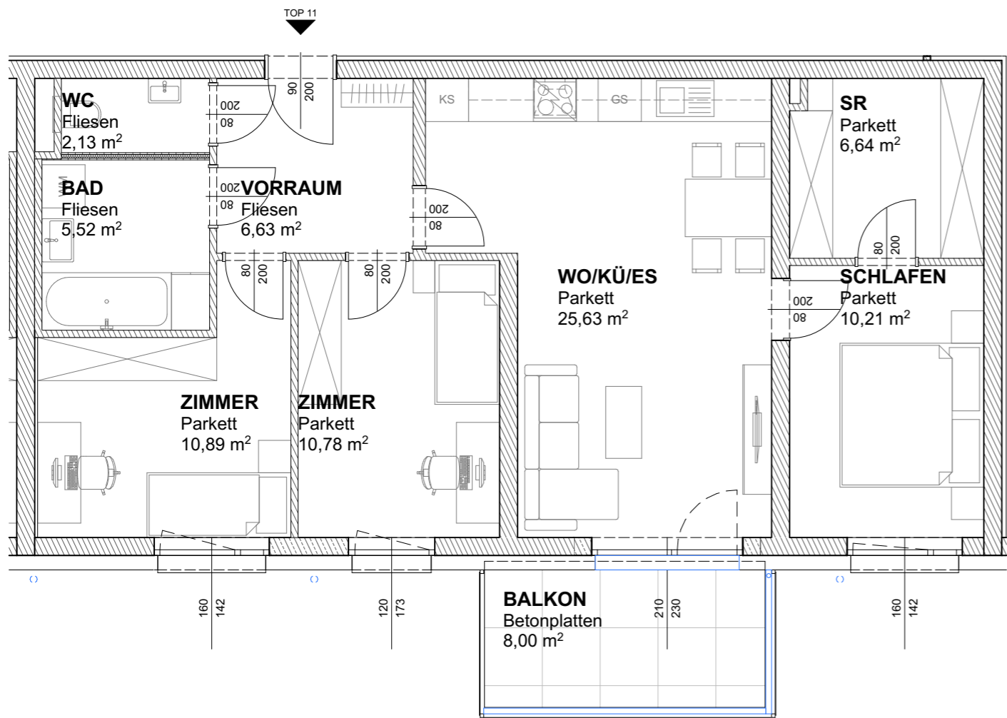
GRUNDRISS | M 1:75
