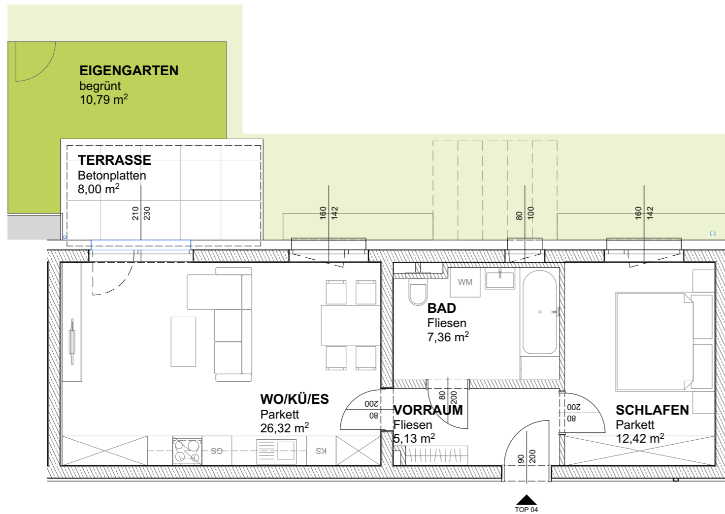
GRUNDRISS | M 1:75
