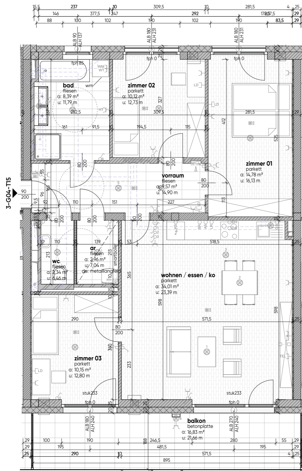
grundriss mit technik M 1:75
