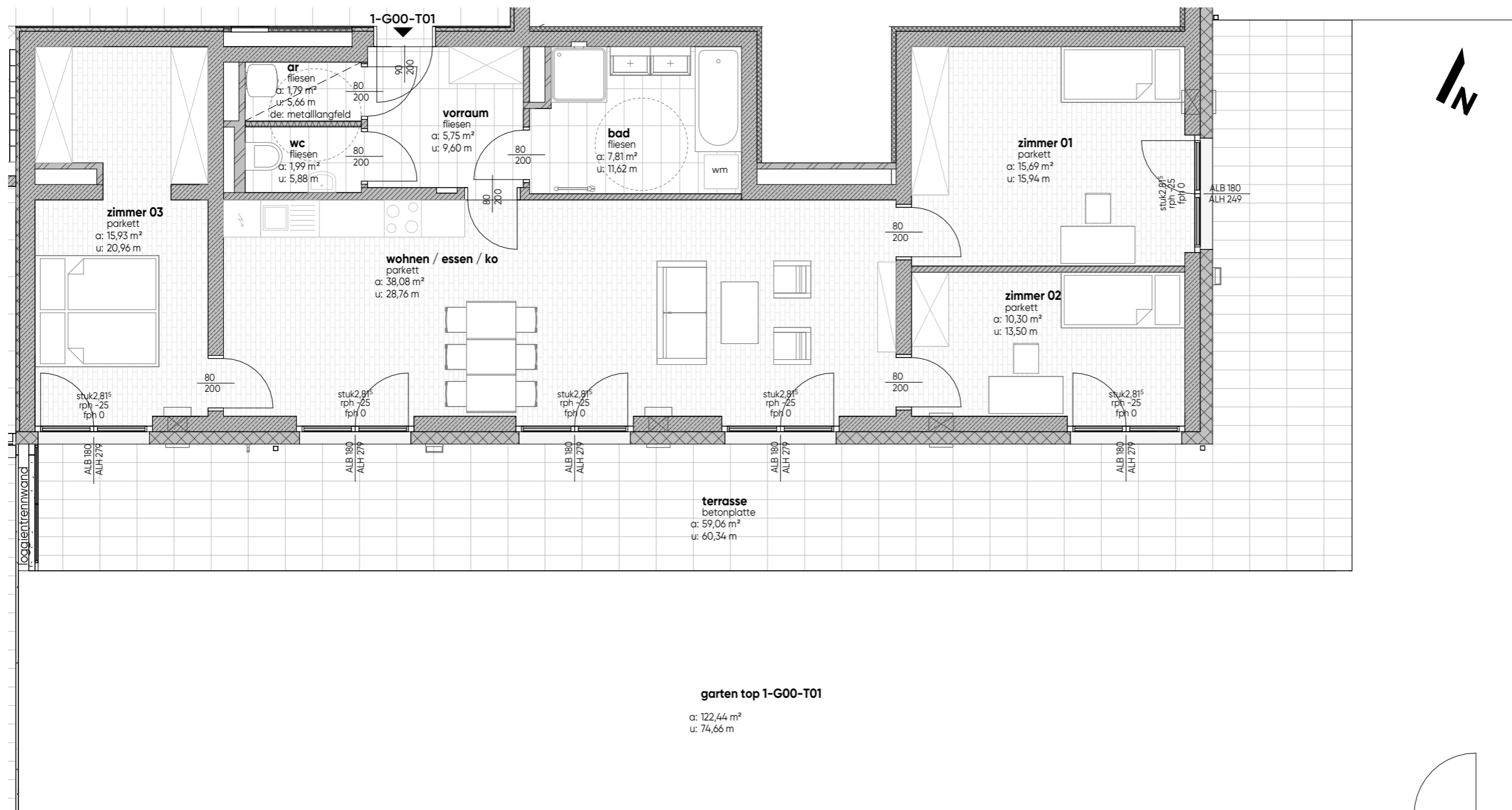
grundriss M1:75
